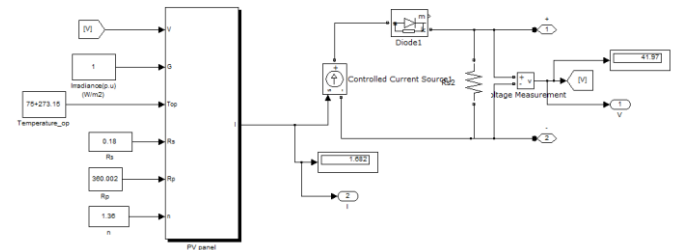
Fig. 13. Simulink Model of PV Module..
